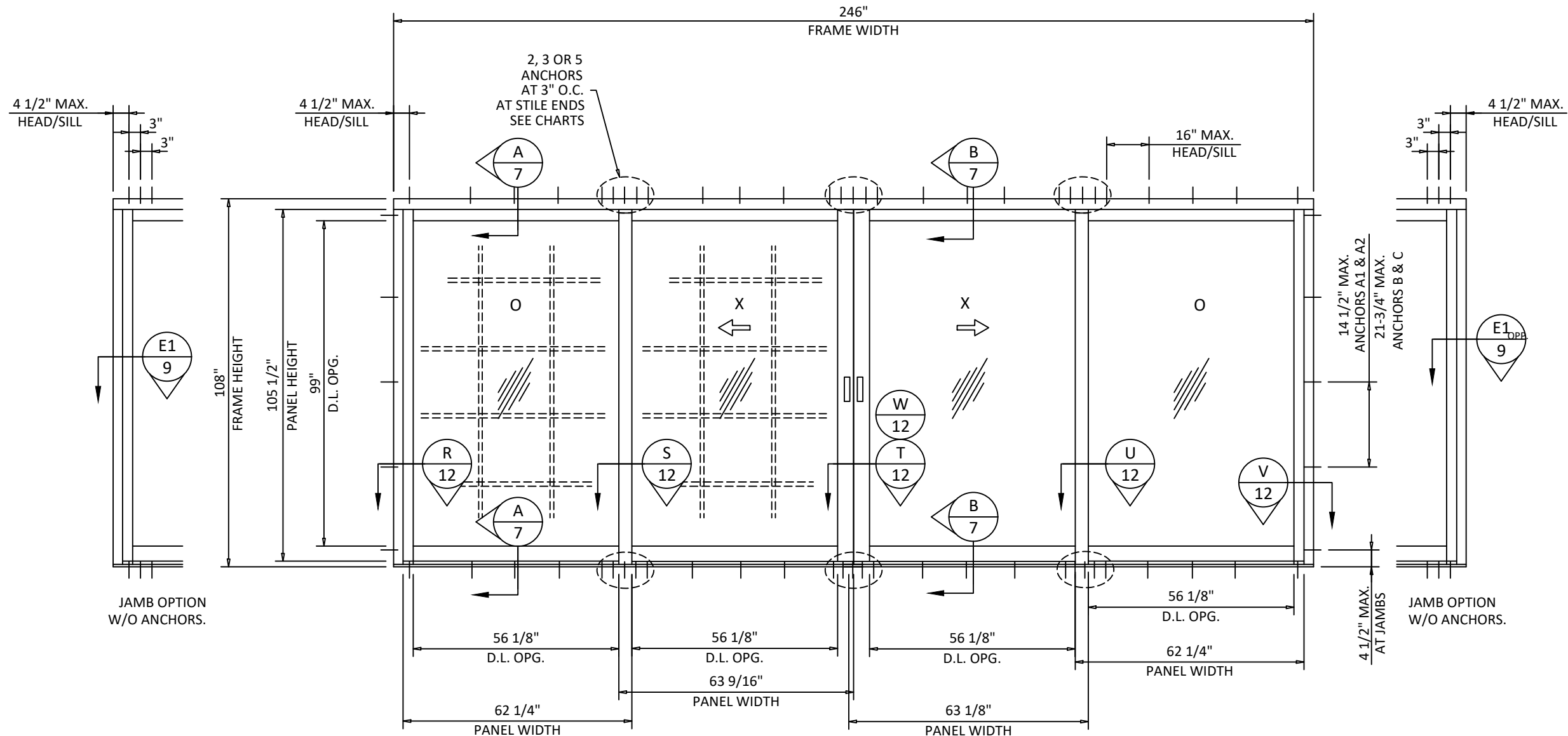
ELEVATION OXXO
